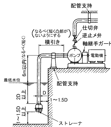
図 2 据付図
