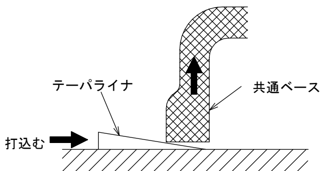
図10 芯出し調整
