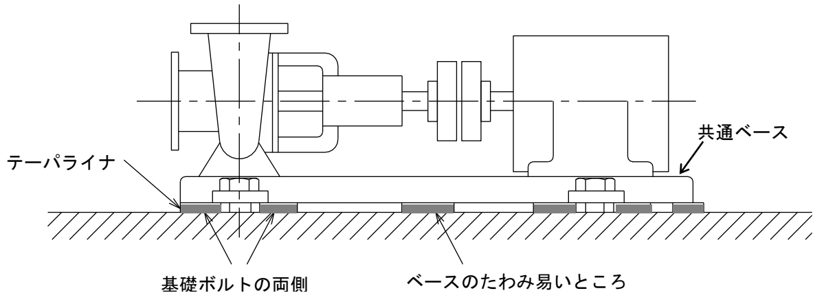
図9 テーパライナ挿入位置
