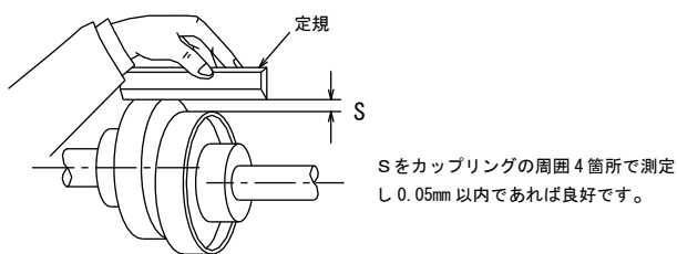
図 4：カップリング外周の段違い
