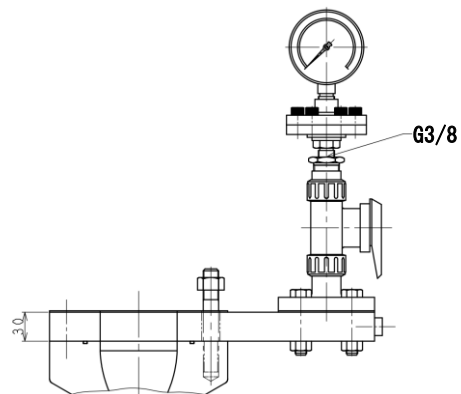
吐出ゲージ用フランジ
