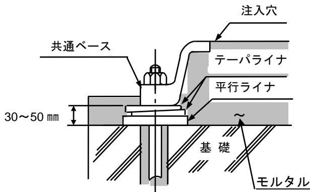
図7：芯出し調整
