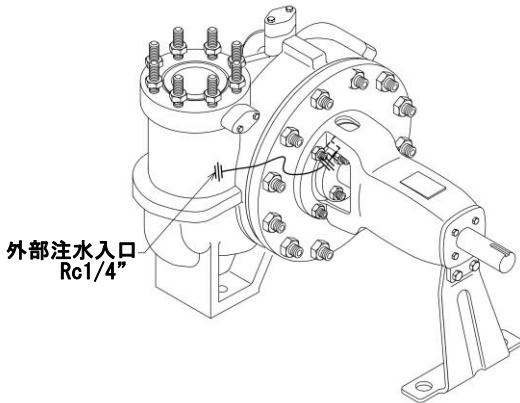
外部注水(グランドパッキンタイプ) 取合いサイズ : Rc-1/4 ユニオン(標準仕様)
