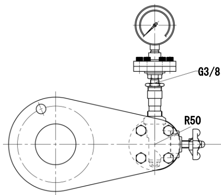
吸込ゲージ用フランジ
