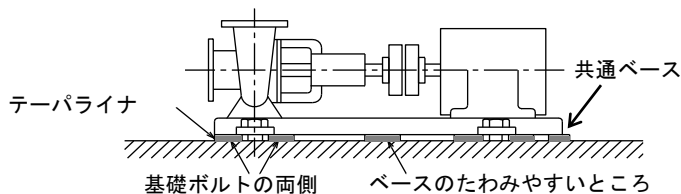
図 6：テーパライナ挿入位置
