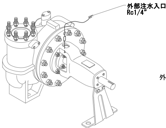
取合いサイズ : Rc-1/4 ユニオン(標準仕様)
