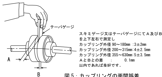
図 5：カップリングの面間誤差
