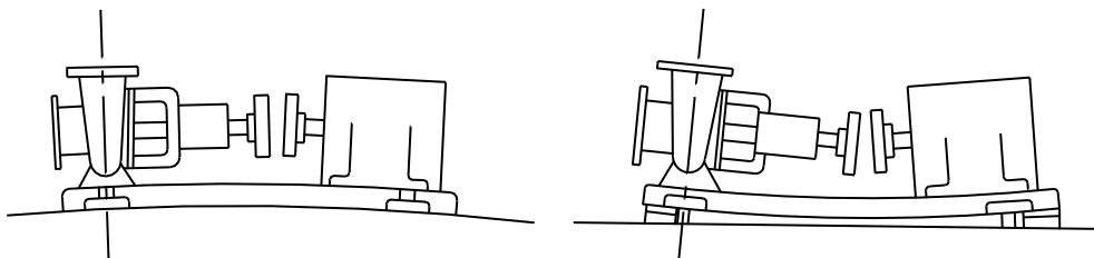
図 3：据付時の軸芯のずれ
