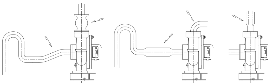
自吸運転不良の起る配管例
