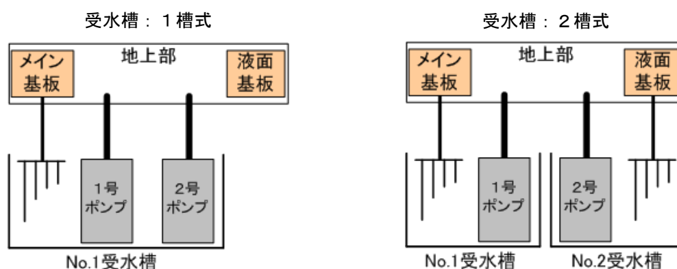
図 11 受水槽とポンプの関係
