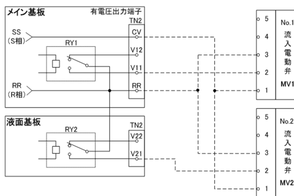
図 9 電動弁 配線パターン 2
