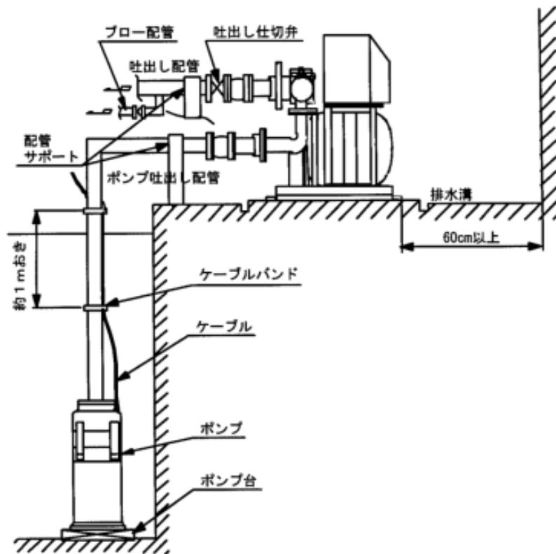
図1 ユニット据付例
