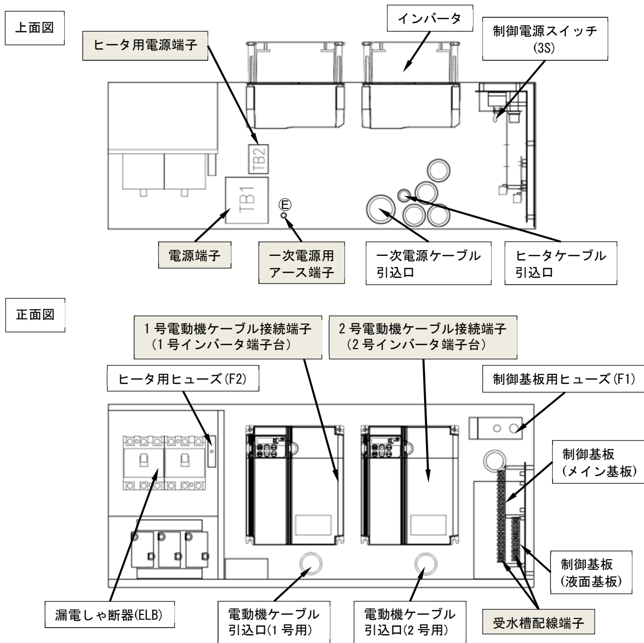
図 4 制御盤内図 3.7kW 以上 (制御盤カバーを外した状態)
