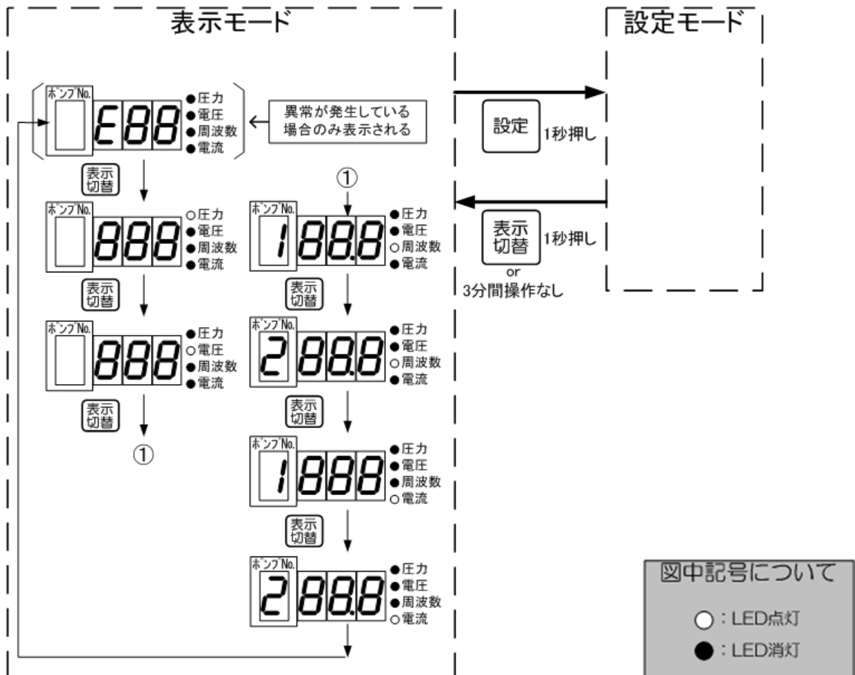
図 27 表示モードの操作方法
