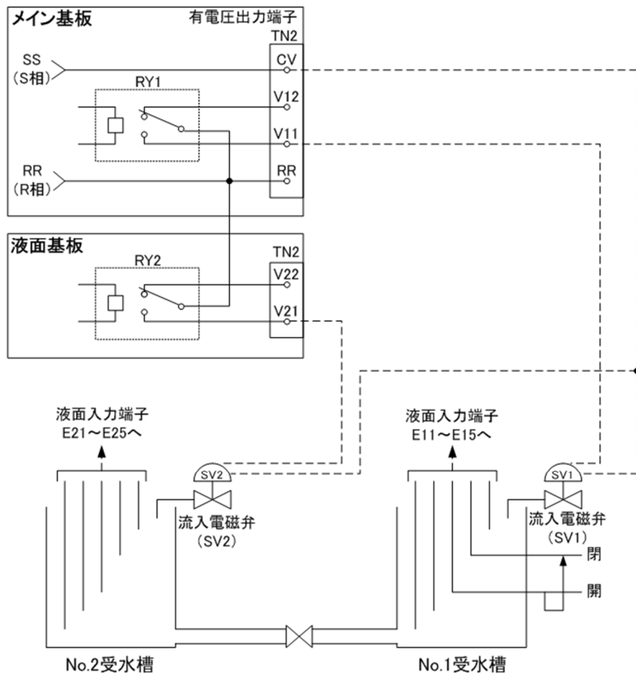
図6 流入電磁弁（通電時開）
