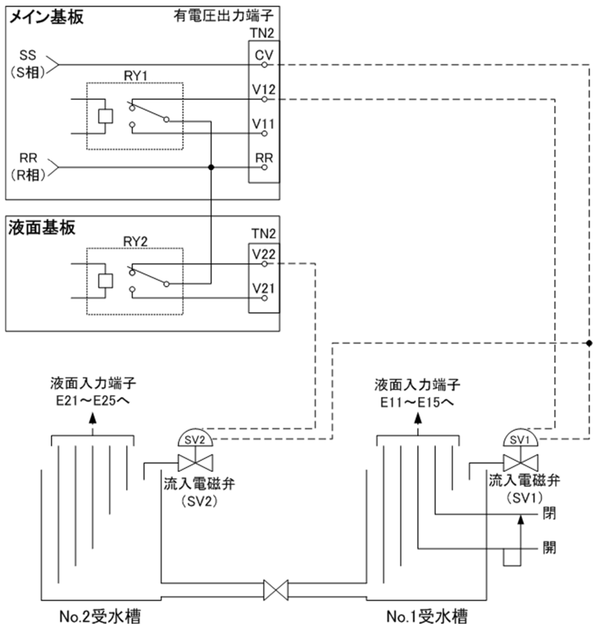
図7 流入電磁弁（通電時閉）
