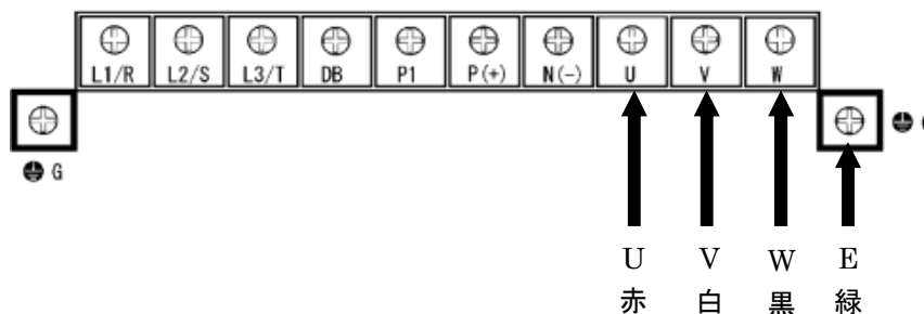
図 5 モーターケーブルの配線方法
