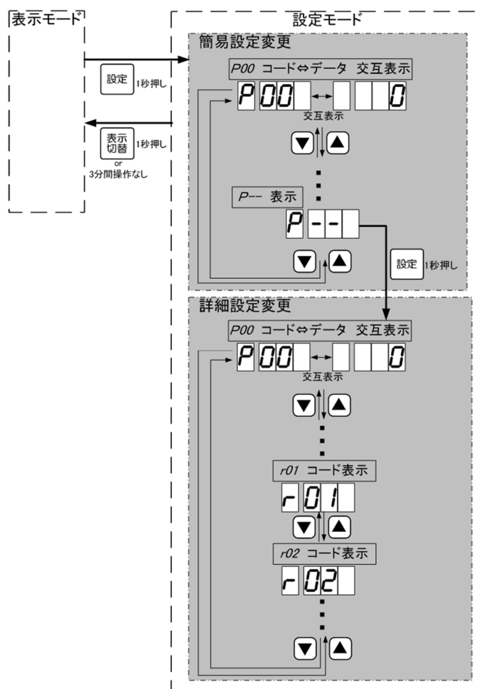
図 35 設定モード内のコード r01 と r02
