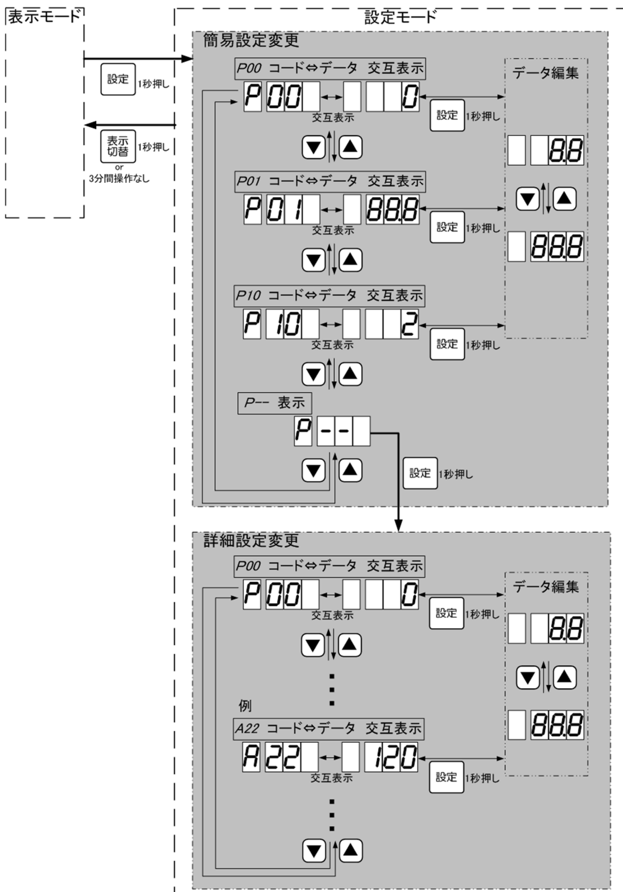
図 28 設定モードの操作方法
