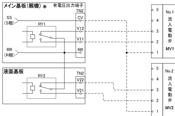
図 9 電動弁 配線パターン 1
