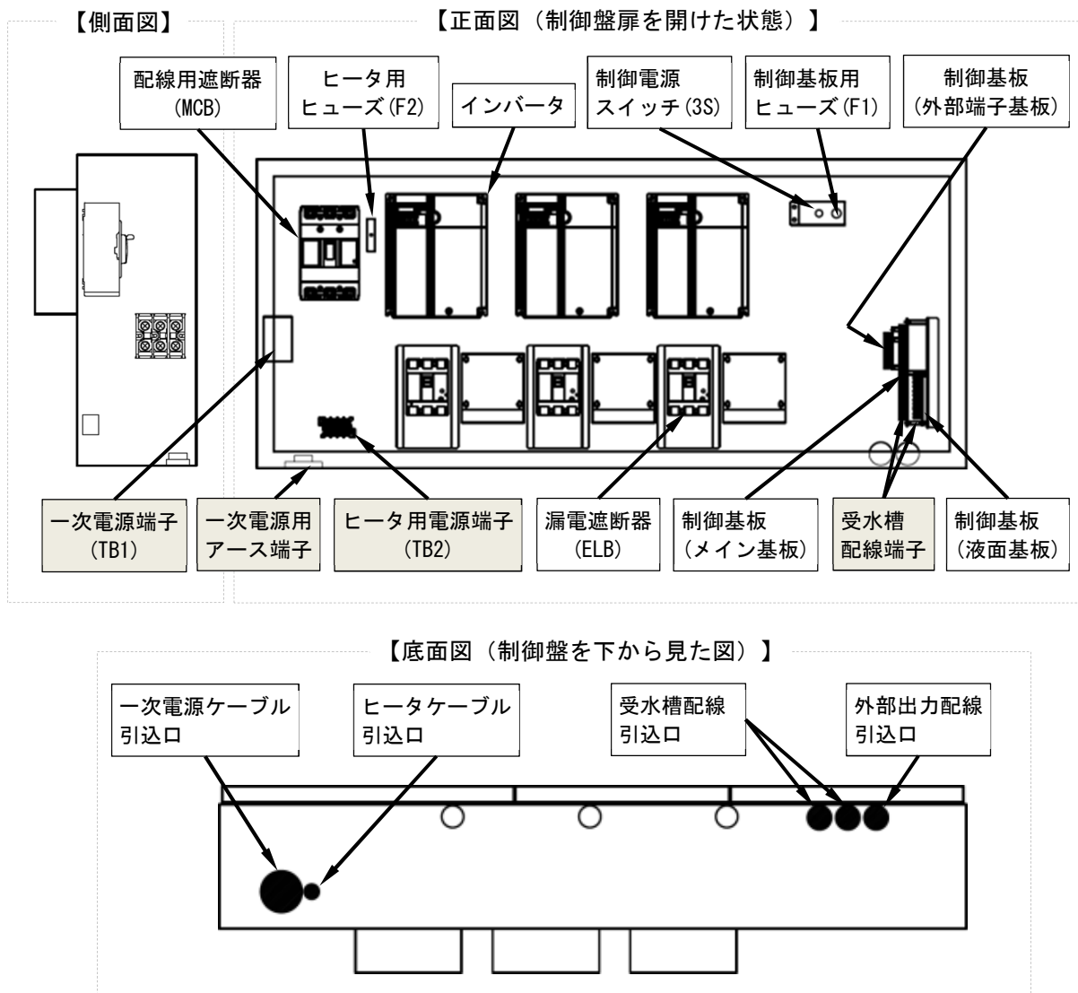
図 6 制御盤 内部配置図
