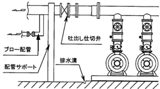
図4 ユニット据付例（吐出し配管）
