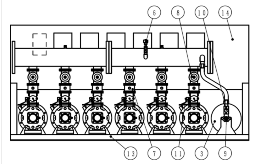
[BNWME/BNYME 型]
