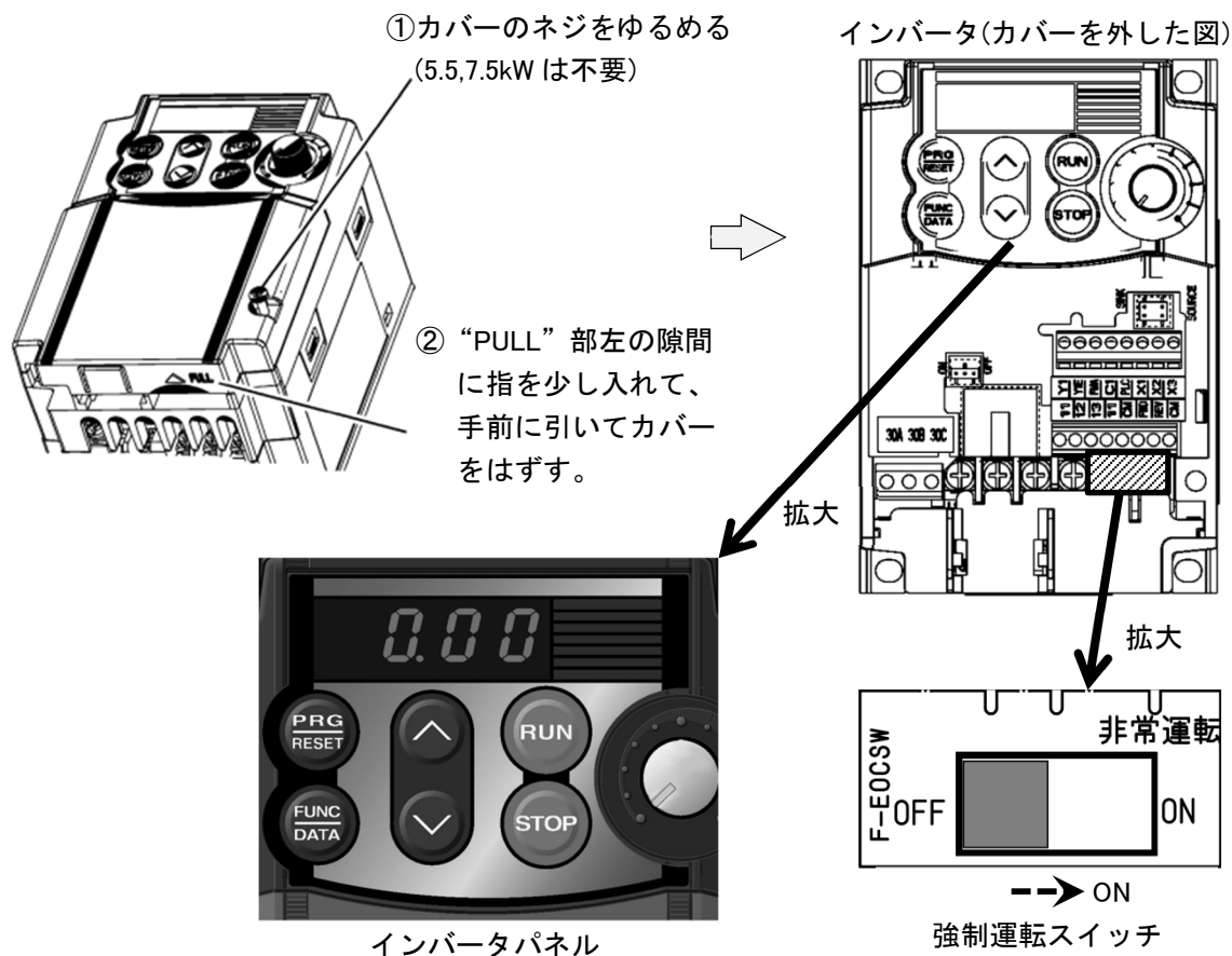
図 39 非常時手動バックアップ運転方法
