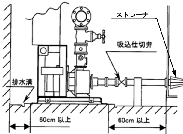
図1 ユニット据付例（流し込みの場合）
