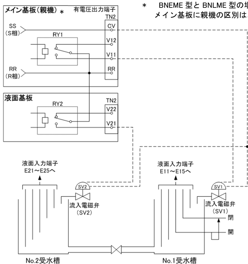
図7 流入電磁弁（通電時開）
