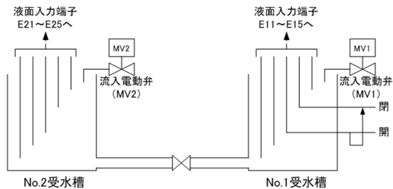
図 11 受水槽側 (配線パターン 1、2 共通)
