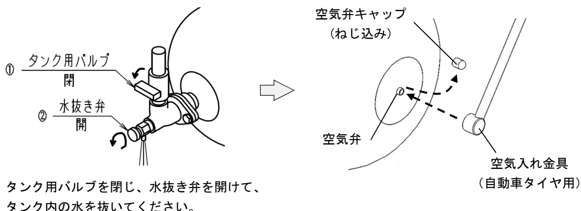
図 40 圧力タンクの空気充填方法
