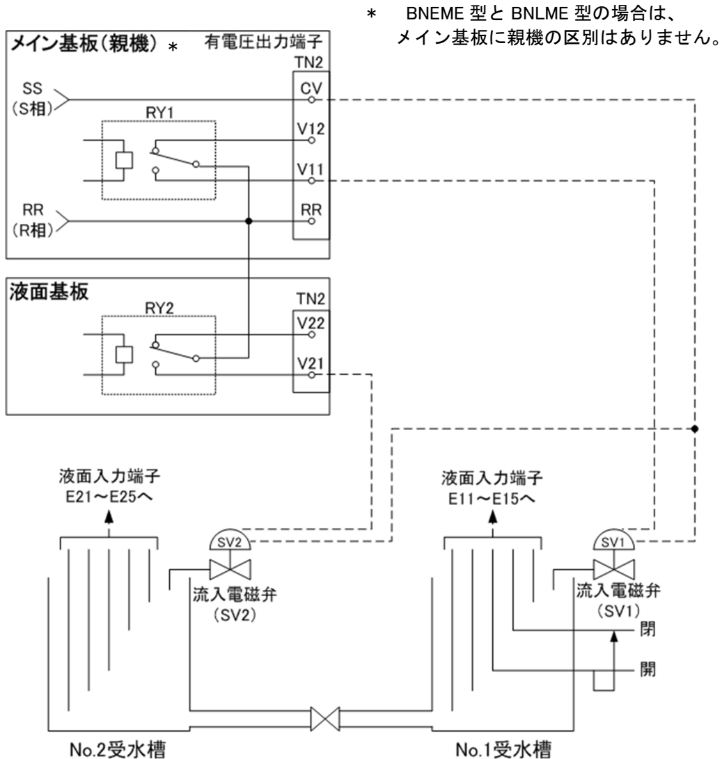
図8 流入電磁弁（通電時閉）
