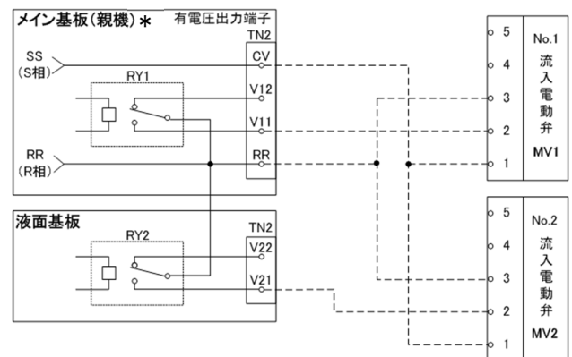
図 10 電動弁 配線パターン 2
