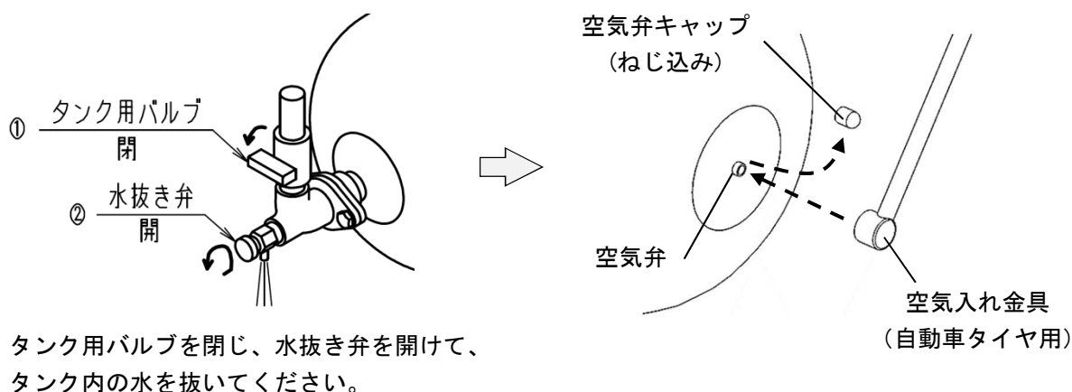
図 38 圧力タンクの空気充填方法
