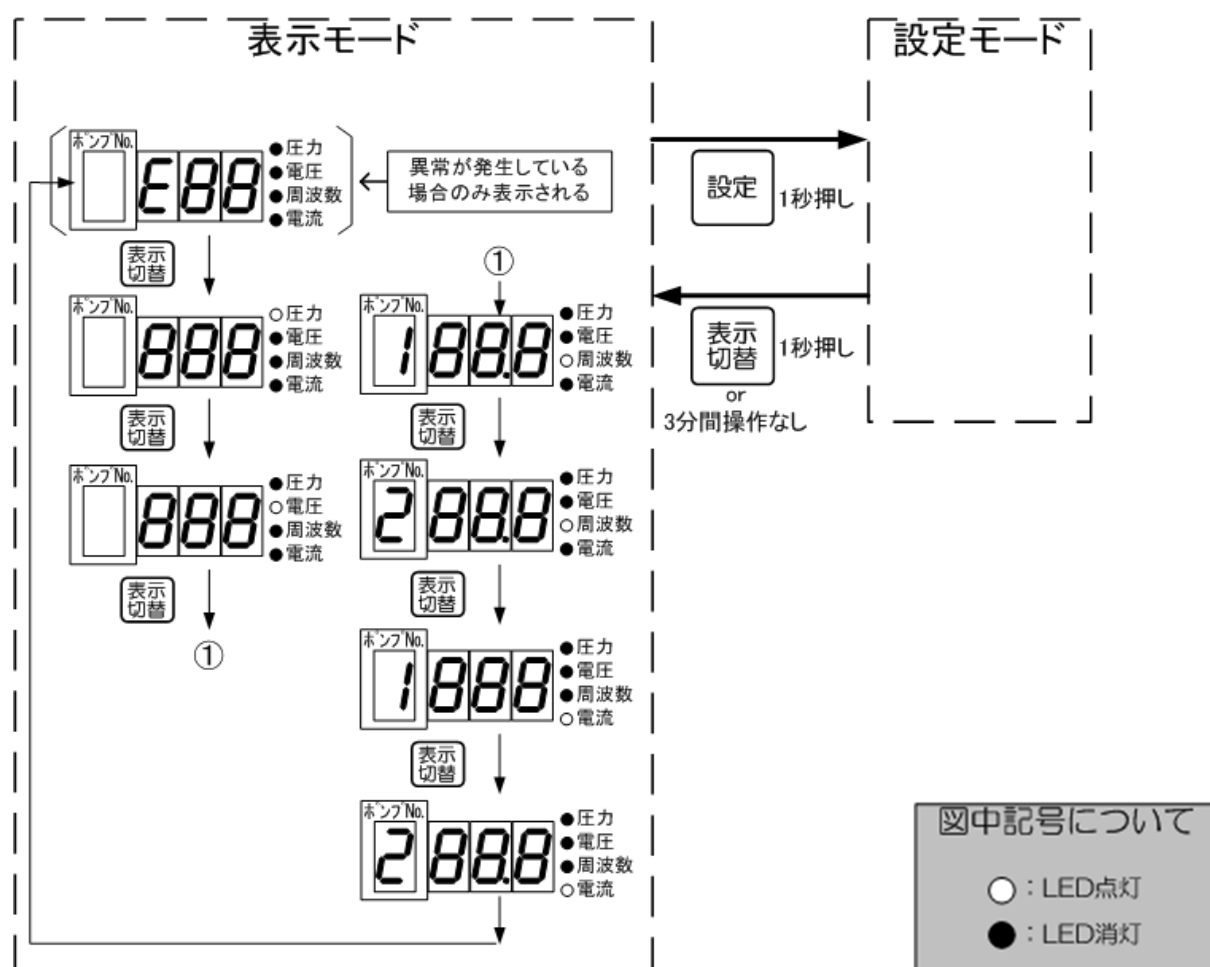
図26 表示モードの操作方法
