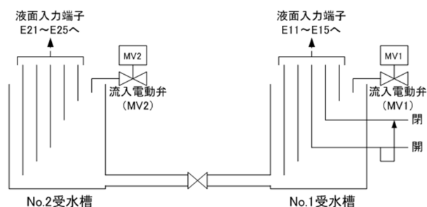
図 10 受水槽側 (配線パターン 1、2 共通)
