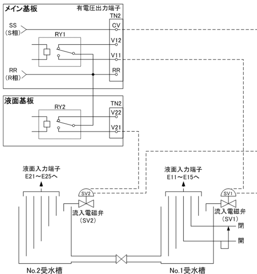
図6 流入電磁弁（通電時開）
