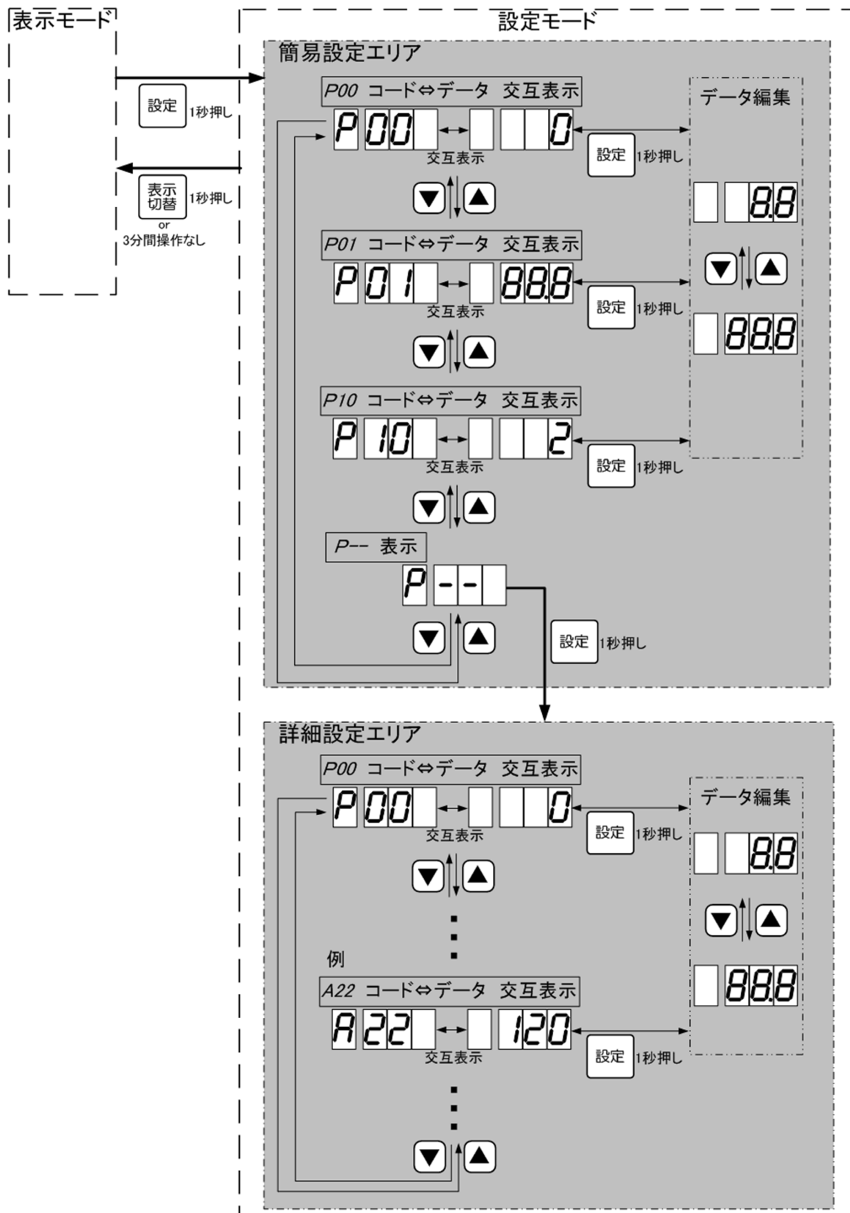
図 27 設定モードの操作方法
