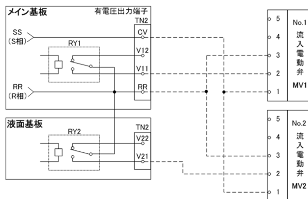
図 9 電動弁 配線パターン 2
