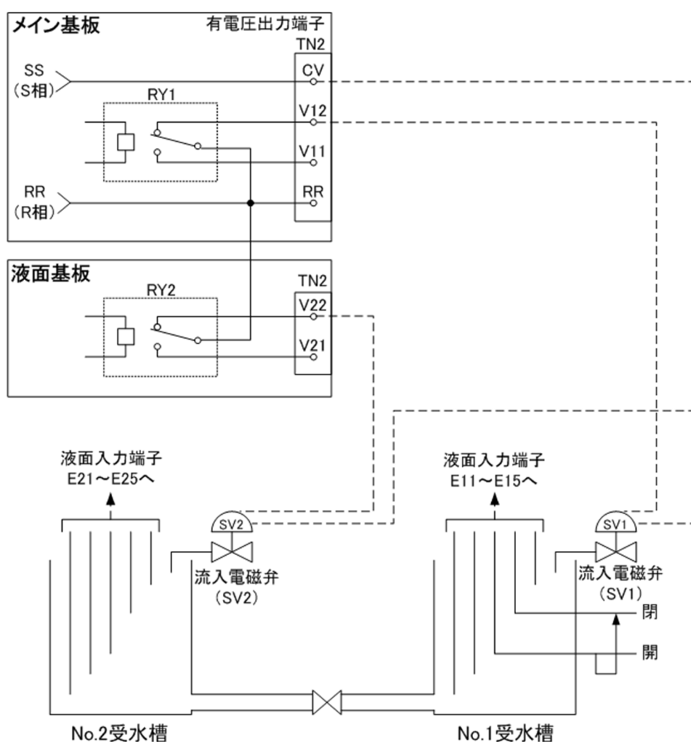
図 7 流入電磁弁（通電時閉）
