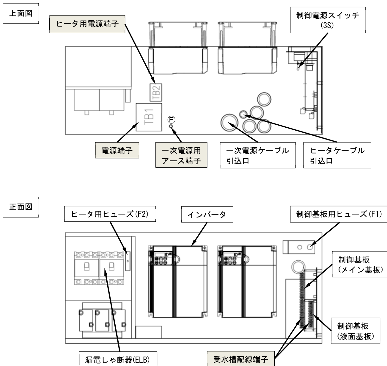
図 5 制御盤内図 5.5kW 以上（制御盤カバーを外した状態）
