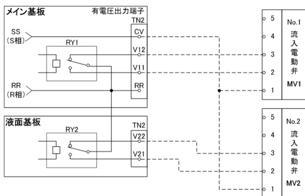
図 8 電動弁 配線パターン 1
