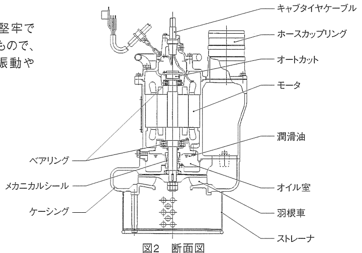
図2 断面図
