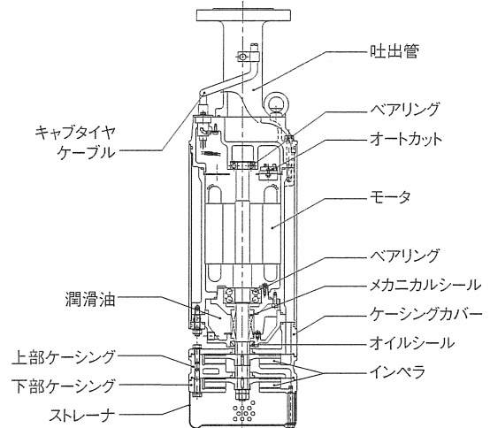
図2 断面図
