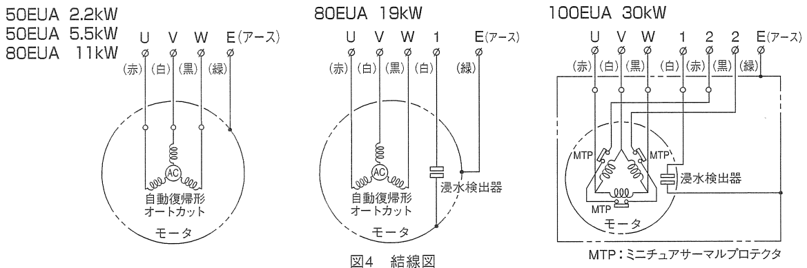
図4 結線図
