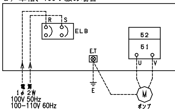
a) 単相、100V級の場合
