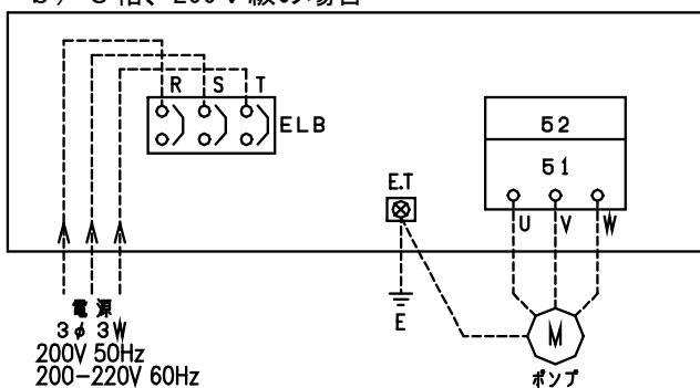
b) 3相、200V級の場合
