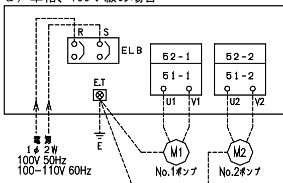
a) 単相、100V級の場合
