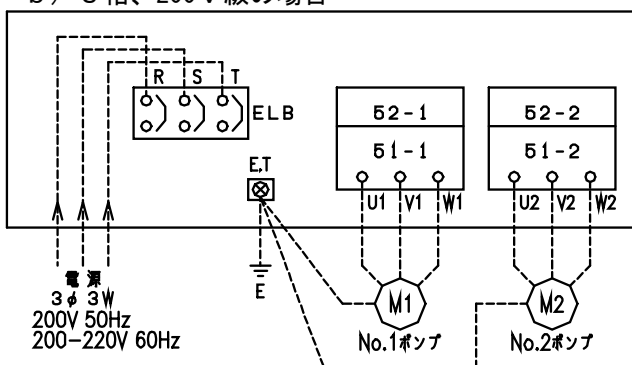
b) 3相、200V級の場合
