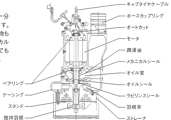
図2 断面図
