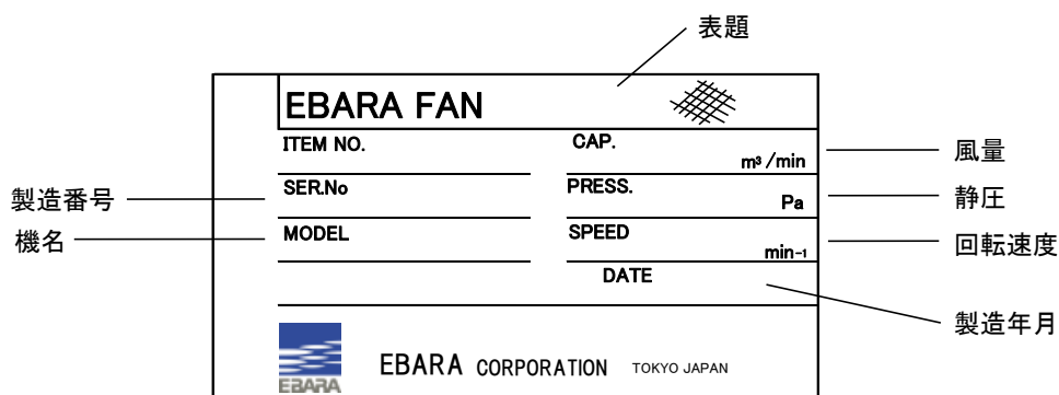
図 1 銘板図
