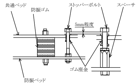
図 6 ストッパーボルト取付(例)
