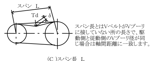
(C)スパン長 L 図 10 Vプーリの心出し
