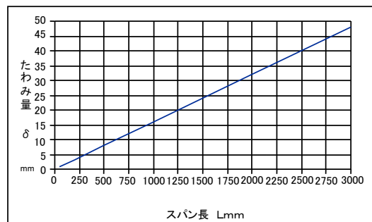
図 12 Vベルトの必要たわみ量 ( \delta mm)
