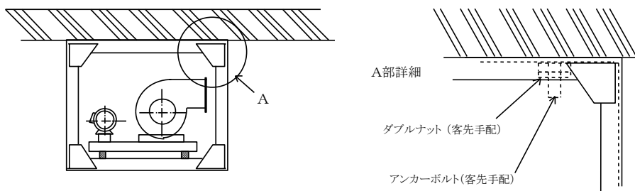
図 8 籠形天井吊り取付(例)
