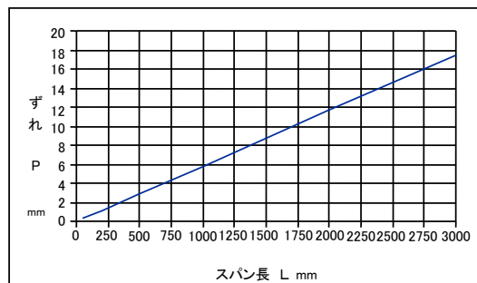
図 11 Vプーリのずれ許容寸法 (Pmm)
