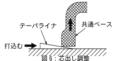
図6：芯出し調整
