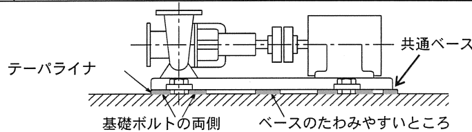
図5：テーパライナ挿入位置
