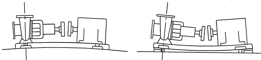
図2：据付時の軸芯のずれ
