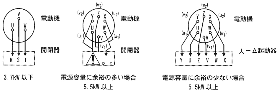
図7：配線接続図
