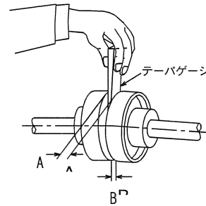
スキミゲージ又はテーパゲージにてA及びBを上下左右で測定し A及びB : 2~4mm AとBとの差 : 0.1mm以内 であれば良好です。 図4：カップリングの面間誤差
