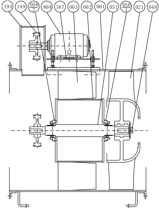
Vベルト駆動型 (No.4 1/2~No.9 AIR2型)
