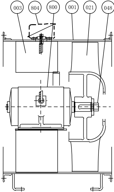
直動型 (No.5~No.11 AIM2型)
