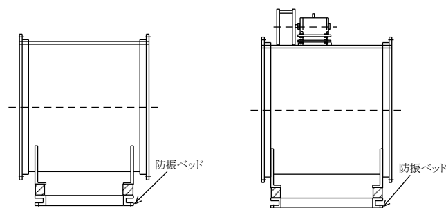
A I M 2 型 A I R 2 型 図 2 床置型 (例)
