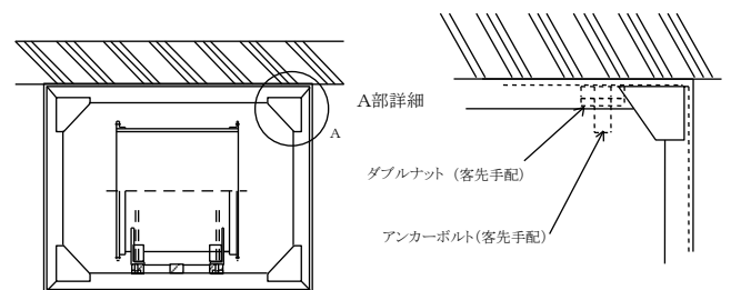
図 8 AIM2型 籠形天井吊り取付 (例)
