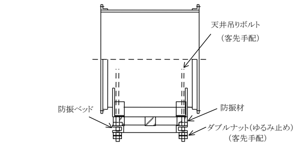
図 5 AIM2型 天井吊り型防振スプリング付 (例)
