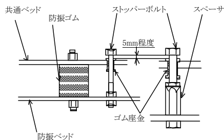
図 6 ストッパーボルト取付(例)
