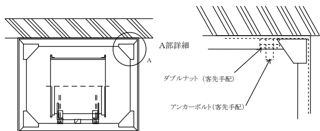
図 8 AIM2型 籠形天井吊り取付 (例)
