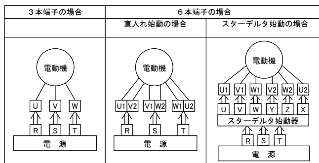
図14 結線図
