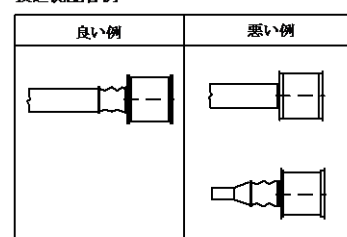
吸込側配管例
