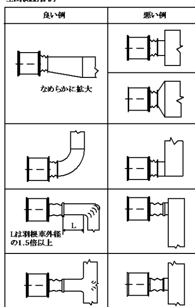
吐出側配管例
