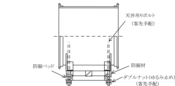
図 5 AIM2型 天井吊り型防振スプリング付 (例)
