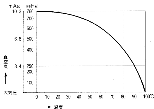
水の蒸発温度と真空度
