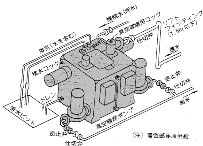
配管例 (AC2K)
