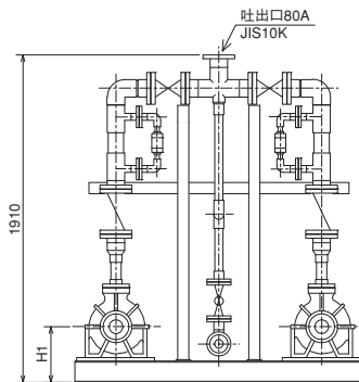
立面図
