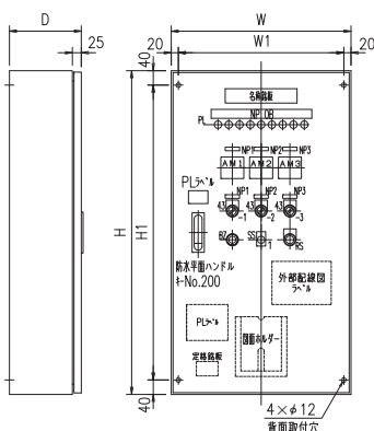
EWR型 3台タイプ外形寸法図
