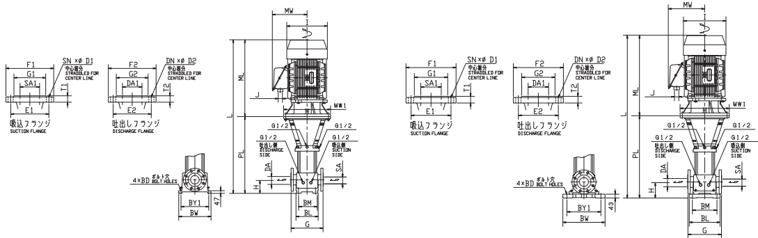
100EVML-R・EVMG-R・EVM-R型
